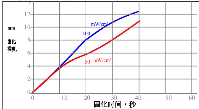
固化设备: Fusion D 灯
